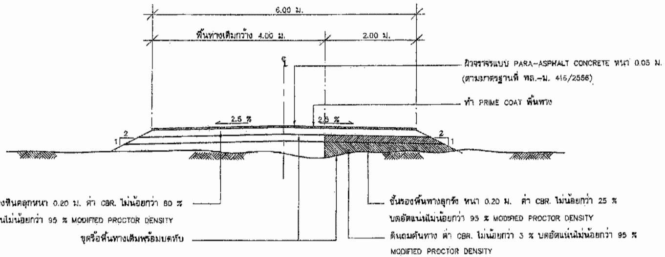
รูปตัดโครงสร้างทางมิวจราจแบบ PARA-ASPHALT CONCRETE กม.0+000 - กม.0+163 และ กม.2+392 - กม.2+490
