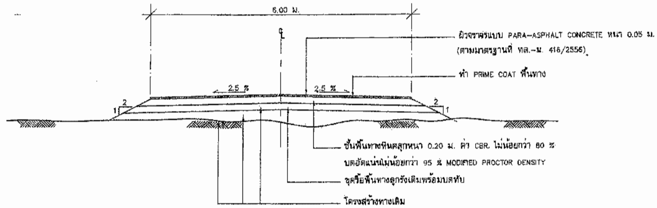
รูปตัดโครงสร้างทางมิวจราจแบบ PARA-ASPHALT CONCRETE กม.0+000 - กม.0+163 และ กม.2+392 - กม.2+490
